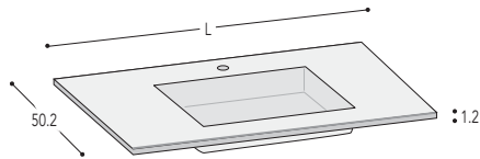
Type 3E - Basin 70 x 31 x 10 Prof. N.B. - ONLY on 90/105/120 L. washbasin units Typ 3E - Becken 70 x 31 x 10 Prof. N.B. NUR auf WT - Unterschränke B.90/105/120
