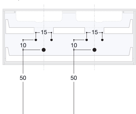
Drains position / Abläufemassen
