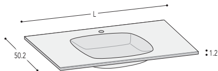
Type 3H - Basin 58 x 32 x 13 Prof. Typ 3H - Becken 58 x 32 x 13 Prof.
