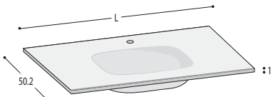
Top type 2F (big rectangular) Basin 75 x 32 x 12 Prof. N.B.- ONLY on 90/105/120 L. washbasin units Platte Typ 2F (rechteckig gross) Becken 75 x 32 x 12 Prof. N.B. NUR auf WT - Unterschränke B.90/105/120
