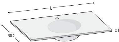
Top type 2H (ellipse) Basin 57 x 30 x 12 Prof. Platte Typ 2H (ekliptisch) Becken 57 x 30 x 12 Prof.
