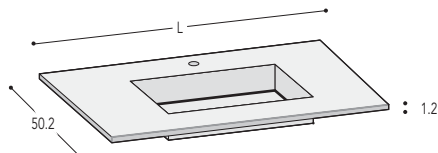
Type 5B (rectangular) Basin 64.5 x 32 x 12 Prof. N.B. - ONLY on 90/105/120 L. washbasin units Typ 5B - (rechteckig) Becken 64.5 x 32 x 12 Prof. N.B. NUR auf WT - Unterschränke B.90/105/120
