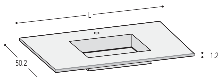
Type 5A (rectangular) Basin 54.5 x 32 x 12 Prof. Typ 5A (rechteckig) Becken 54.5 x 32 x 12 Prof.
