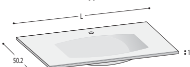
Top type 2L (soft big) Basin 65 x 32 x 12 Prof. N.B.- ONLY on 90/120 L. washbasin units Platte Typ 2L (soft gross) Becken 65 x 32 x 12 Prof. N.B. NUR auf WT - Unterschränke B.90/120
