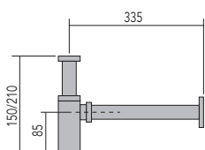
siphon QUADRATO Siphon viereckig
