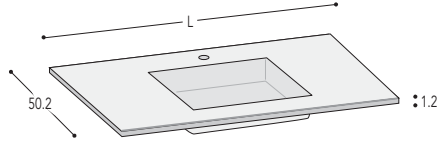
Type 3D - Basin 60 x 31 x 10 Prof. N.B. - ONLY on 90/105/120 L. washbasin units Typ 3D - Becken 60 x 31 x 10 Prof. N.B. NUR auf WT - Unterschränke B.90/105/120
