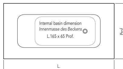
Bathtub "PROJECT" H.52 Capacity Kg 322 Badewanne "PROJECT" H.52 Kapazität Kg 322
