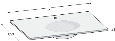
Top type 2G (eye) Basin 64 x 30 x 12 Prof. N.B.- ONLY on 90/105/120 L. washbasin units Platte Typ 2G (Augen) Becken 64 x 30 x 12 Prof. N.B. NUR auf WT - Unterschränke B.90/105/120
