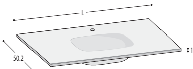
Top type 2D (small rectangular) Basin 57 x 32 x 12 Prof. Platte Typ 2D (rechteckig klein) Becken 57 x 32 x 12 Prof
