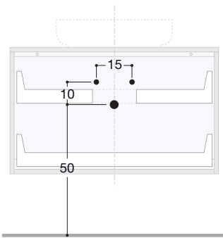
Drains position / Abläufmassen
