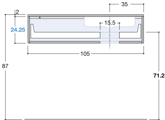
Drains position / Abläufmassen
