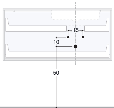
Drains position / Abläufemassen
