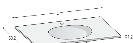
Type 3I - Basin 79 x 34 x 13 Prof. N.B. - ONLY on 90/105/120 L. washbasin units Typ 3I - Becken 79 x 34 x 13 Prof. N.B. NUR auf WT - Unterschränke B.90/105/120
