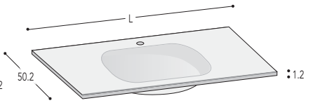
Type 3Q - Basin 74 x 35,7 x 12,5 Prof. N.B. - ONLY on 90/105/120 L. washbasin units Typ 3Q - Becken 74 x 35,7 x 12,5 Prof. N.B. NUR auf WT - Unterschränke B.90/105/120
