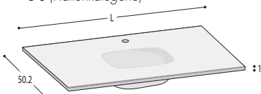
Top type 2C (rectangular) Basin 49 x 31 x 12 Prof. Platte Typ 2C (rechteckig) Becken 49 x 31 x 12 Prof.
