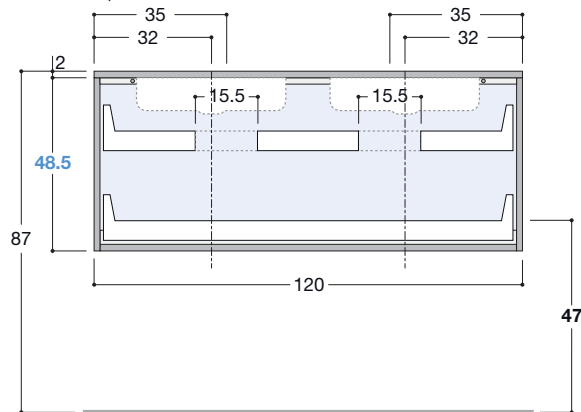
Drains position / Abläufemassen
