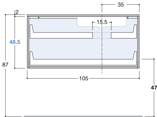
Drains position / Abläufemassen
