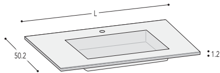
Type 3S - Basin 90 x 31 x 10 Prof. N.B. - ONLY on 105/120 L. washbasin units Typ 3S - Becken 90 x 31 x 10 Prof. N.B. NUR auf WT - Unterschränke B.105/120
