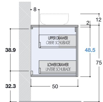
Side view D.50 / Seitenansicht T.50
