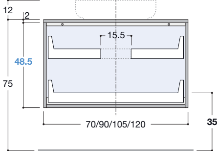
Drains position / Abläufmassen
