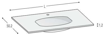
Type 3F - Basin 75 x 34 x 13 Prof. N.B. - ONLY on 90/105/120 L. washbasin units Typ 3F - Becken 75 x 34 x 13 Prof. N.B. NUR auf WT - Unterschränke B.90/105/120
