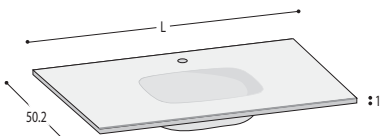
Top type 2E (medium rectangular) Basin 65 x 32 x 12 Prof. N.B.- ONLY on 90/105/120 L. washbasin units Platte Typ 2E (rechteckig medium) Becken 65 x 32 x 12 Prof. N.B. NUR auf WT - Unterschränke B.90/105/120
