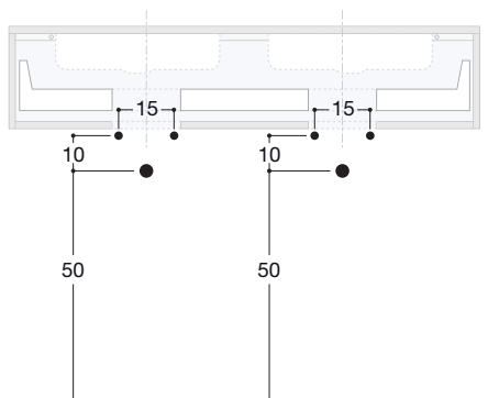
Drains position / Abläufmassen
