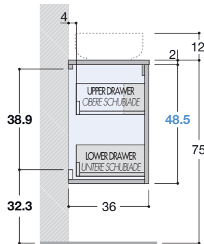
Side view D.36 / Seitenansicht T.36
