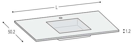
Type 3C - Basin 50 x 31 x 10 Prof. Typ 3C - Becken 50 x 31 x 10 Prof.
