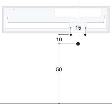
Drains position / Abläufmassen
