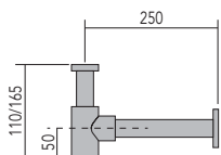
Siphon Round Siphon abgerundet
