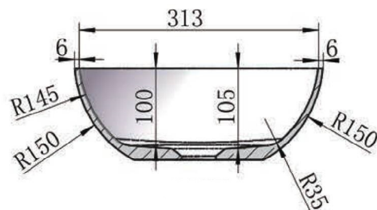
Querschnitt
